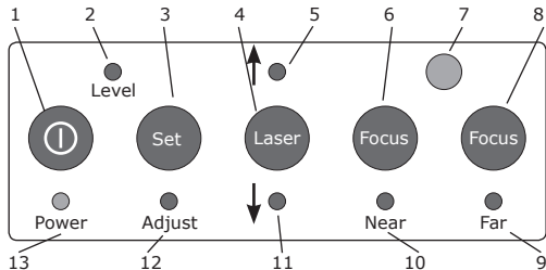
Рис. 3. Панель управления прибором
